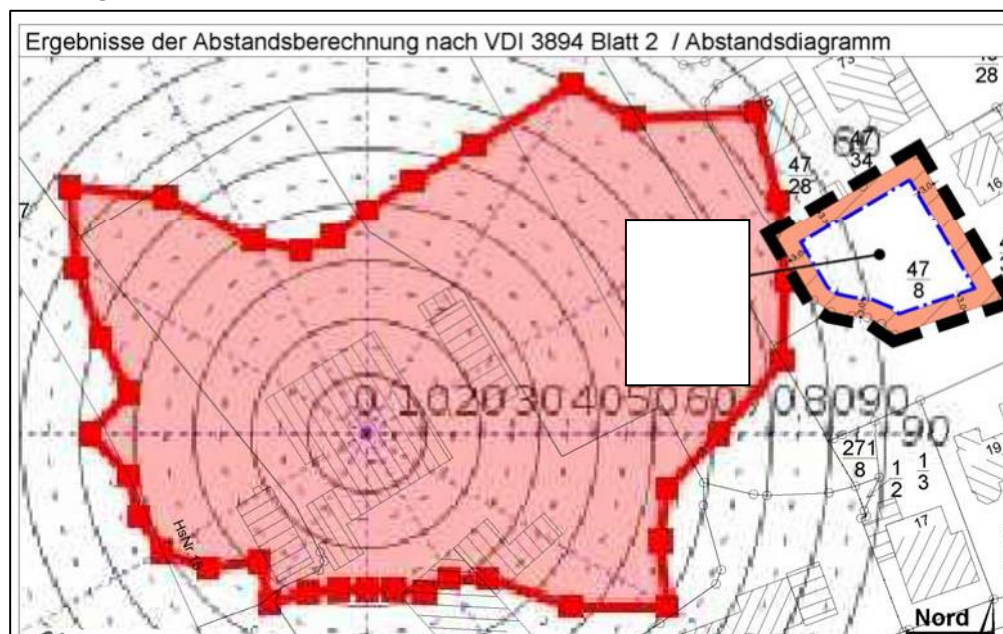
Abb. 6: Ergebnis der Abstandsberechnung nach VDI 3894 / Abstandsdigramm Geruchshäufigkeit (ohne Maßstab)
