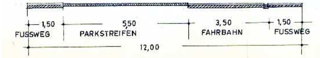
STRASSENPROFIL M. 1:100 PLANSTRASSE A
